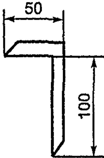
Рисунок А.3 - Шаблон для измерения профиля горки
